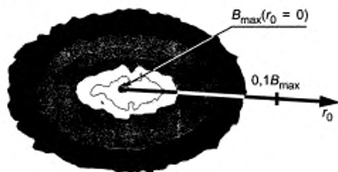
Рисунок С.1 — Участок повышенной магнитной индукции
