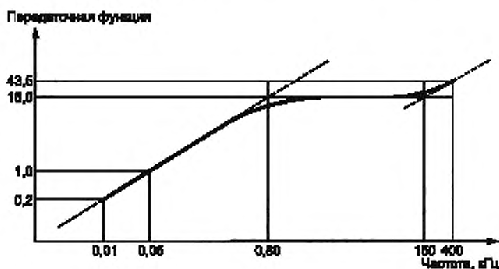
Рисунок 1 — Передаточная функция
