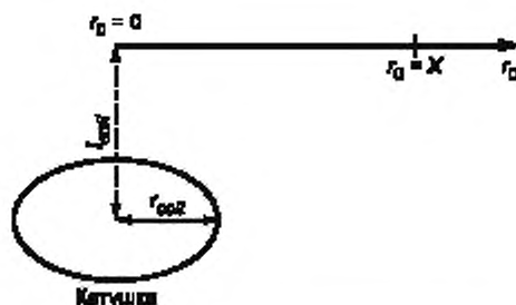
Рисунок С.3 — Расположение эквивалентной катушки
