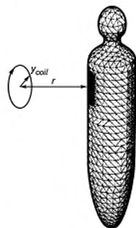
Рисунок Е.2 — Положение источника магнитного поля относительно модели человеческого тела
