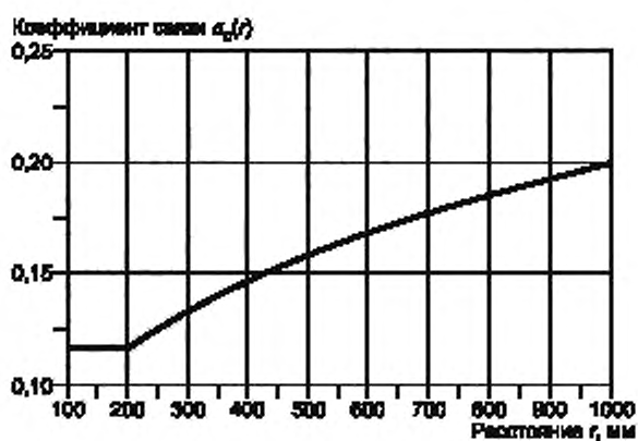
Рисунок С.4 — График зависимости коэффициента связи от расстояния r
