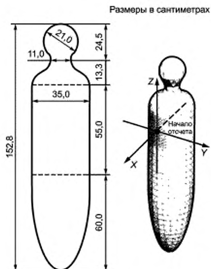
Рисунок Е.1 — Численная модель человеческого тела
