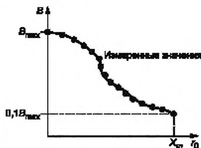
Рисунок С.2 — Градиент магнитной индукции
