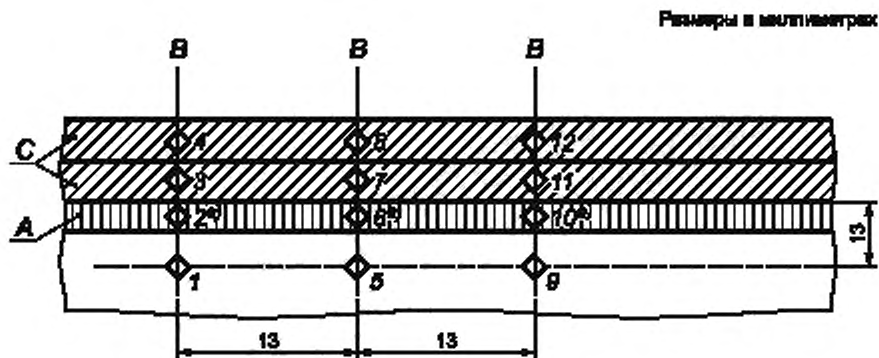
A — зона термического влияния шва (видима после травления); B — линии вдавливаний при анализе твердости (с 1 по 12); C — слой наплавления (видимый после травления).
