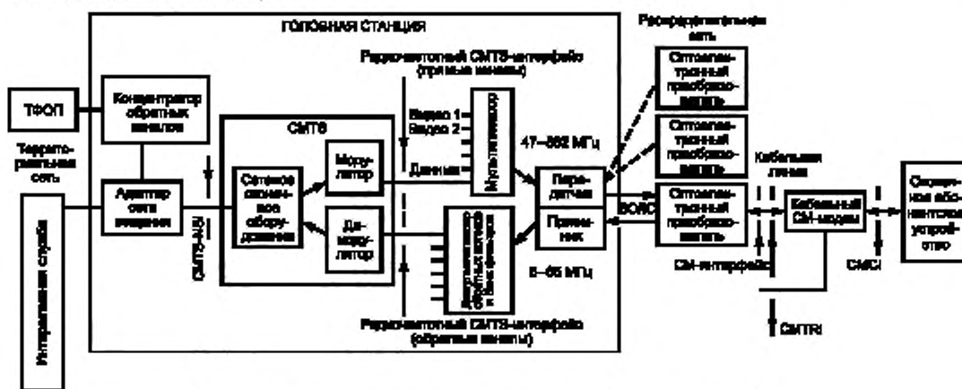
Рисунок 11 — Структурная схема интерактивной системы КТВ J.122
