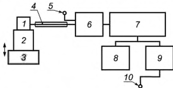
1 — датчик вибрации; 2 — система крепления; 3 — вибрирующая поверхность; 4 — соединительный кабель; 5 — электрический вход; 6 — устройство согласования входного сигнала; 7 — фильтр; 8 — показывающее устройство с устройством выделения и хранения пикового значения; 9 — устройство согласования выходного сигнала; 10 — аналоговый/цифровой выход
