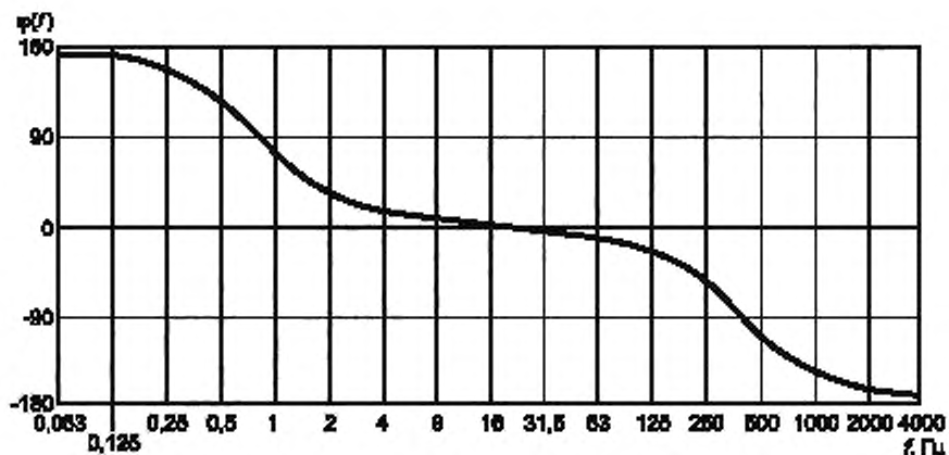
Рисунок 3 — Фазочастотная характеристика измерительной цепи
