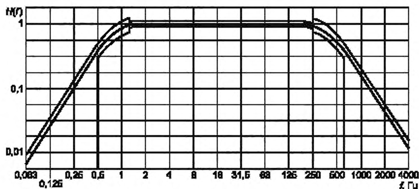
Рисунок 2 — Амплитудно-частотная характеристика измерительной цепи
