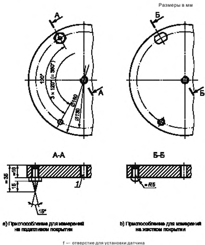
Рисунок 1 — Приспособления для быстрой установки датчиков вибрации
