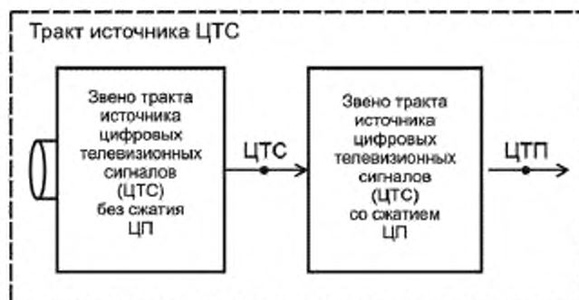
Рисунок 2 — Звенья тракта источника цифровых телевизионных сигналов
