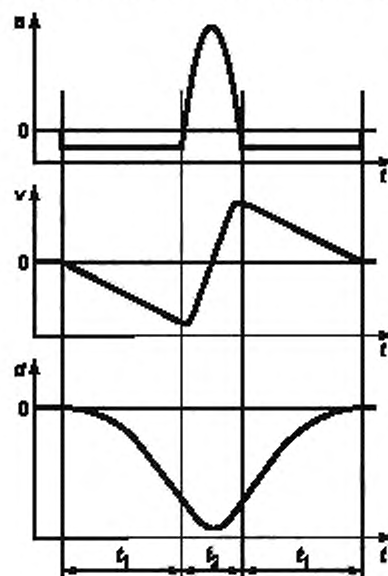
Рисунок С.1 — Сигналы ускорения, скорости и перемещения для импульса полусинусоидальной формы
