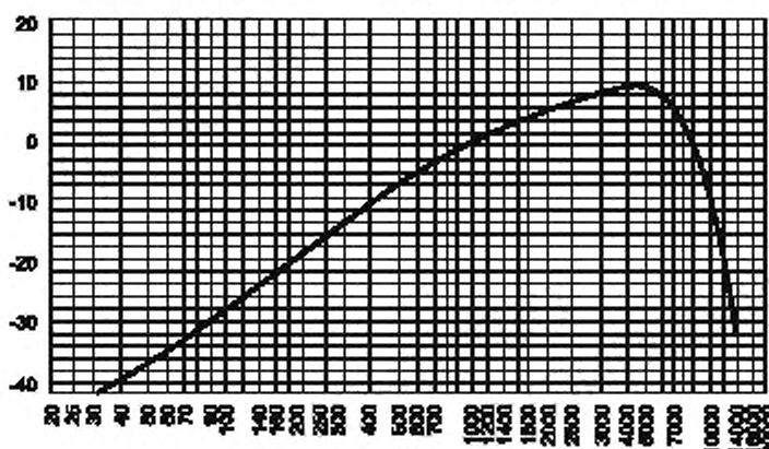
Рисунок 14 — График АЧХ псифометрического фильтра в соответствии с [5]
