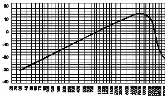
Рисунок 13 — График АЧХ псифометрического фильтра в соответствии с [4]
