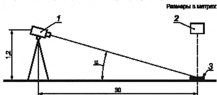
1 — фотоприемник; 2 — источник света типа D 85 по ГОСТ 7721; 3 — поверхность разметки
