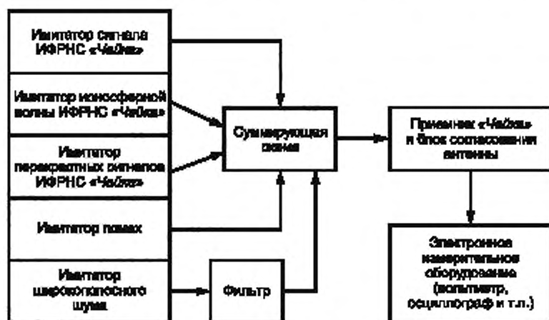
Рисунок 1 — Типовое испытательное оборудование
