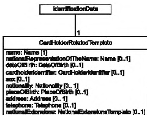
Рисунок 1 — Диаграмма классов на языке UML
