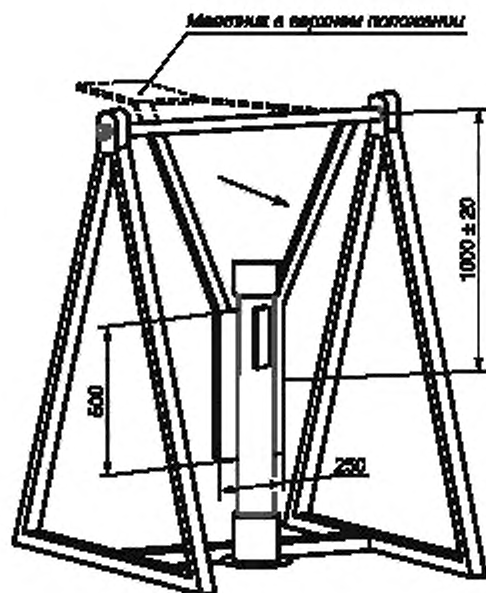
Рисунок 11 — Схема установки маятникового типа
