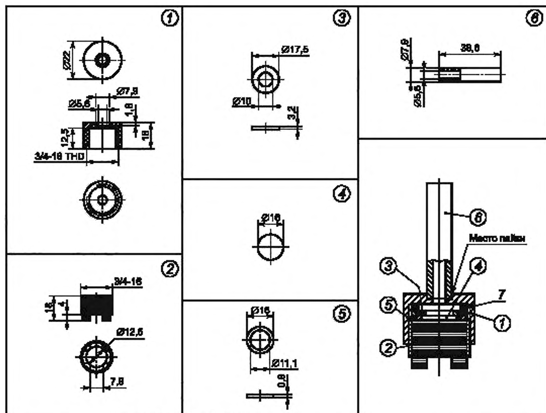
1 — деталь корпуса с внутренней резьбой 3/4-16 THD; 2 — фиксирующая деталь (болт типа 4 с внешней резьбой 3/4-16); 3 — диафрагма; 4 — экран сита номинальным размером 17 × 100; 5 — шайба; 6 — медная трубка; 7 — «O»-образное кольцо наружным диаметром 17,5 мм и внутренним — 12,5 мм
