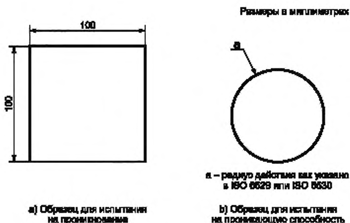
Рисунок 1 — Испытуемые образцы
