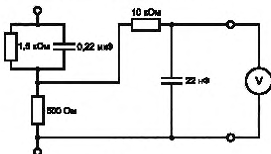
Рисунок 1 — Схема измерения тока прикосновения
