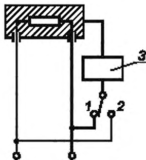
1 и 2 — входные клеммы; 3 — схема по рисунку 1
