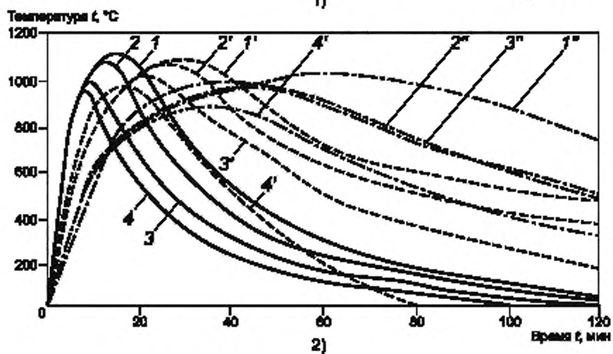
Рисунок 9а — Результаты расчета изменения параметров при объемном пожаре в помещении объемом V = 95 \text{ м}^3 для температур поверхности перекрытия (9а-1) и средневolumной (9а-2) ([5])
