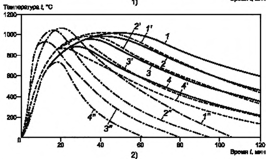
Рисунок 9в — Результаты расчета изменения параметров при пожаре в помещении объемом V = 50,3 \text{ м}^3 для температур поверхности перекрытия (9в-1) и средневolumной (9в-2) ([5])
