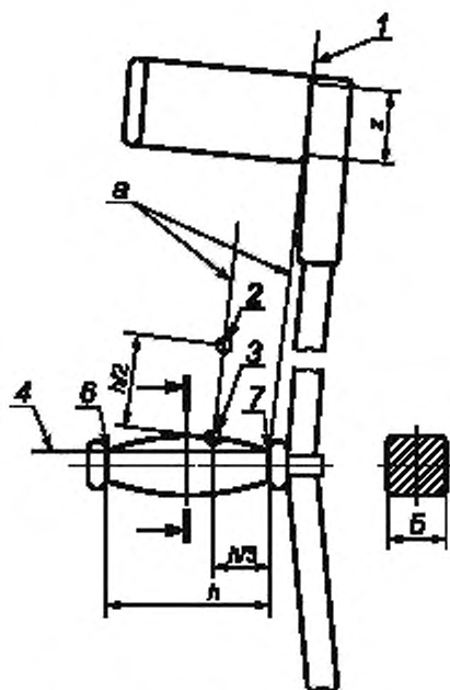
1 — линия опоры манжеты; 2 — точка сустава запястья; 3 — реперная точка; 4 — линия опоры рукоятки; 5 — ширина рукоятки; 6 — передняя контрольная точка рукоятки; 7 — задняя контрольная точка рукоятки; h — длина рукоятки; z — внутренняя высота манжеты
