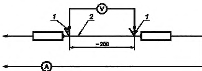
1 — зажимные измерительные щупы. 2 — испытываемая проволока
