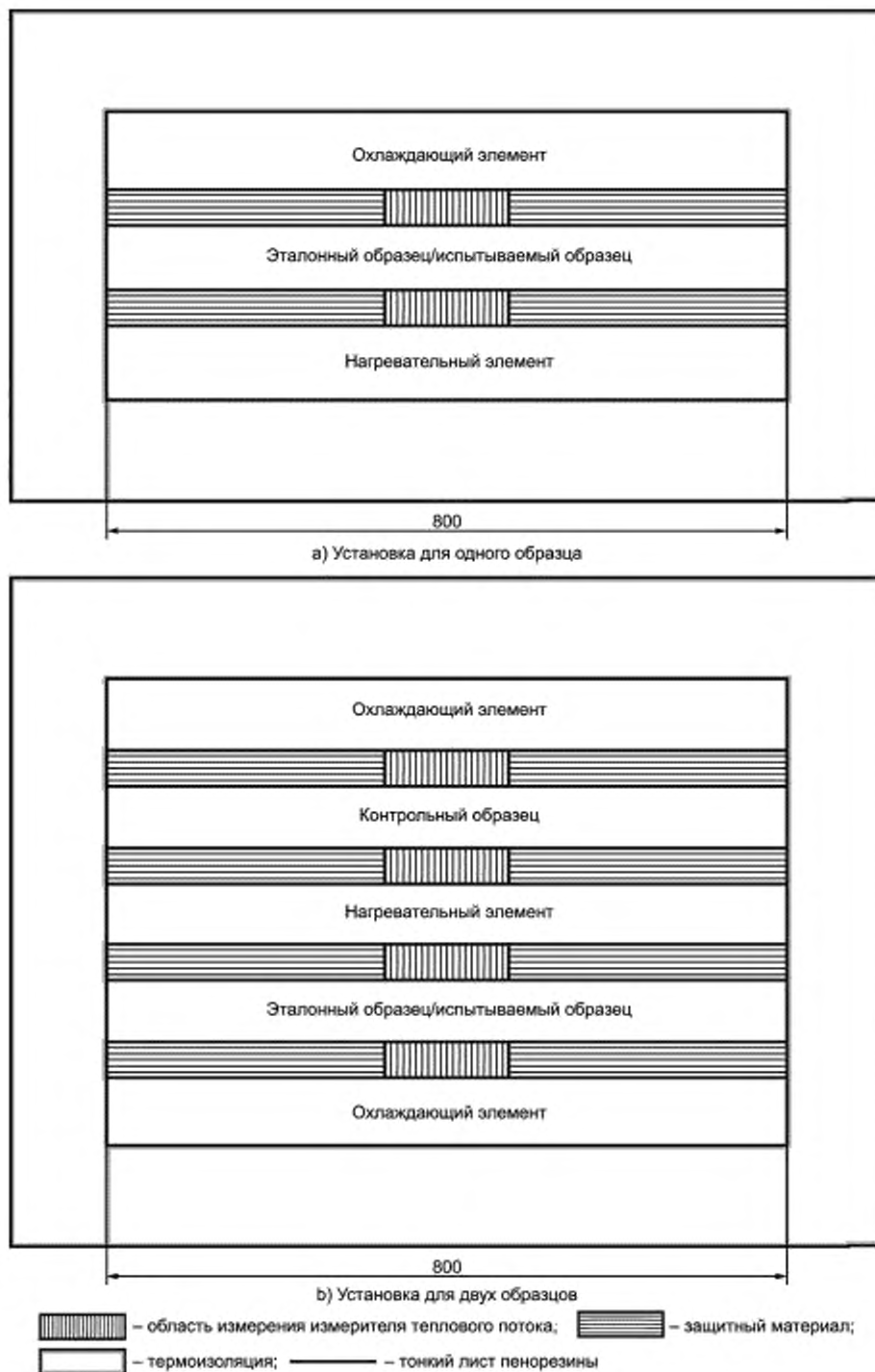
Рисунок 1 — Конфигурация испытательного оборудования
