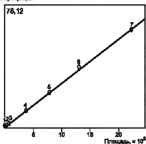
Рисунок 2 — Типичный калибровочный график хлорида
