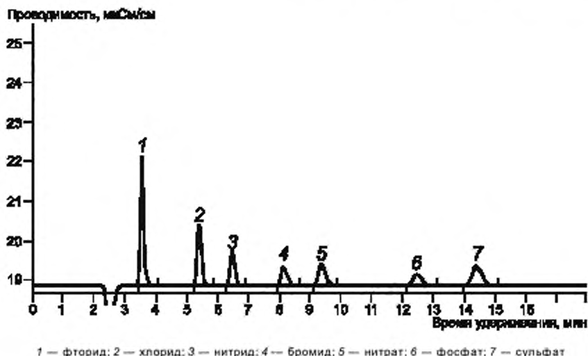
Рисунок 1 — Типовая хроматограмма ионов раствора, содержащая 1 \text{ мг/дм}^3 различных анионов в воде
