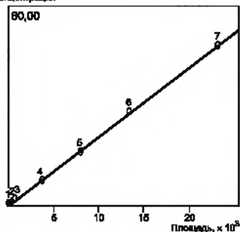
Рисунок 3 — Типичный калибровочный график сульфата
