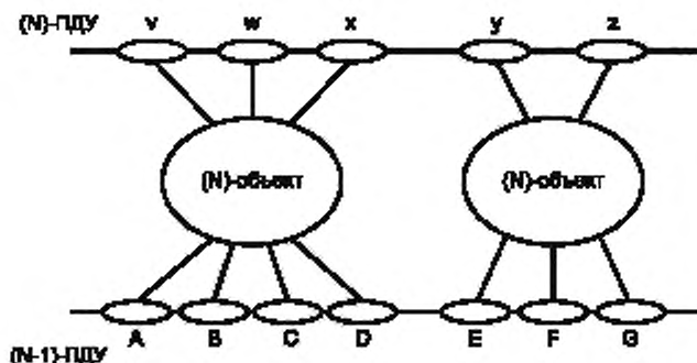
Рисунок 8a — Взаимосвязи между селекторами, относящимися к (N)-ПДУ и (N-1)-ПДУ
