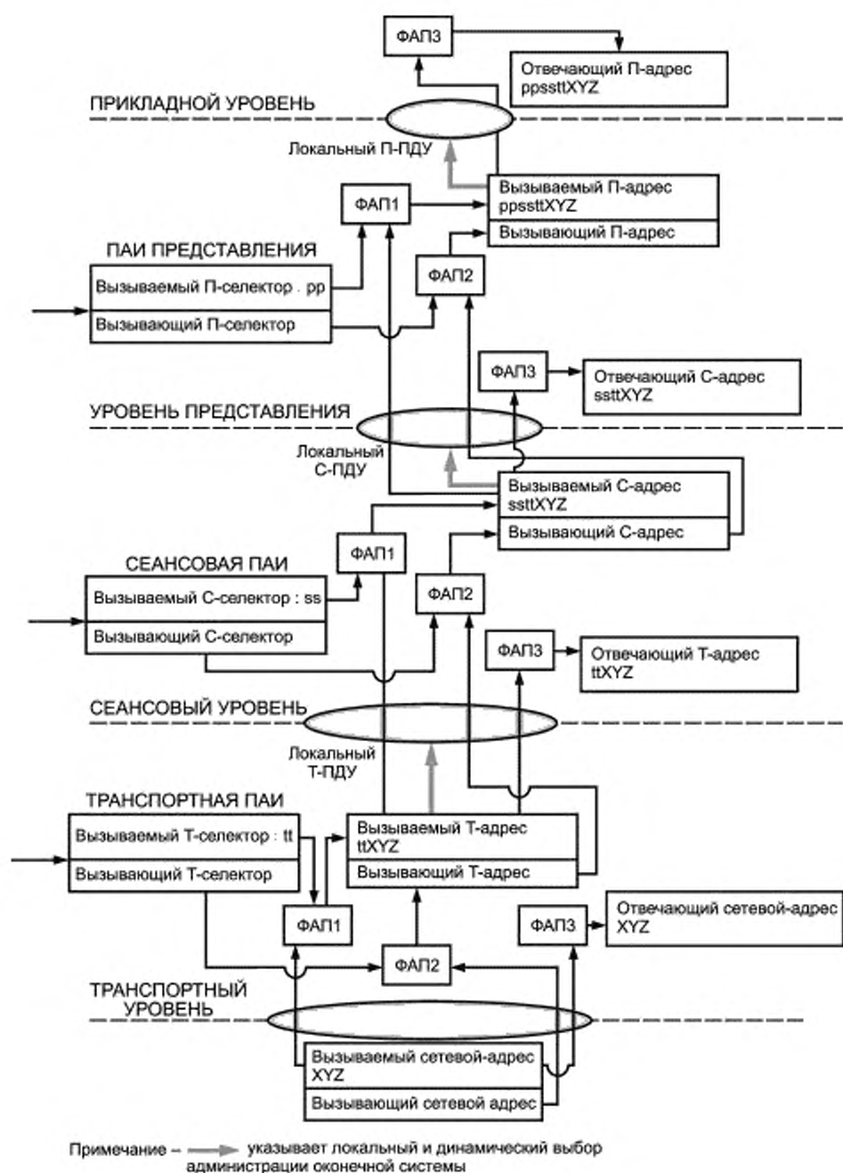
Рисунок 11 — Влияние методов получения в вызываемой оконечной системе
