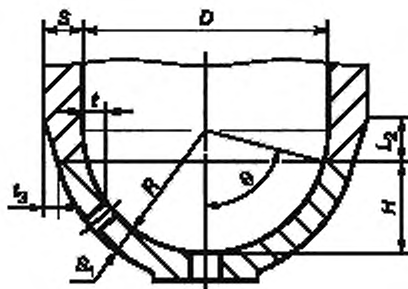
Рисунок 6.5 — Сферическое днище
