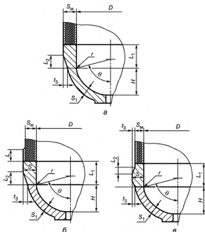
Рисунок 6.8 — Сферические днища с углом сегмента 87^\circ > \theta \geq 75^\circ , сопряженные с многослойной обечайкой посредством вставки
