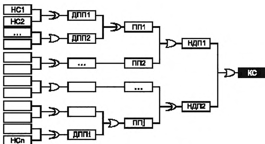
Рисунок 2 — Структура дерева отказов
