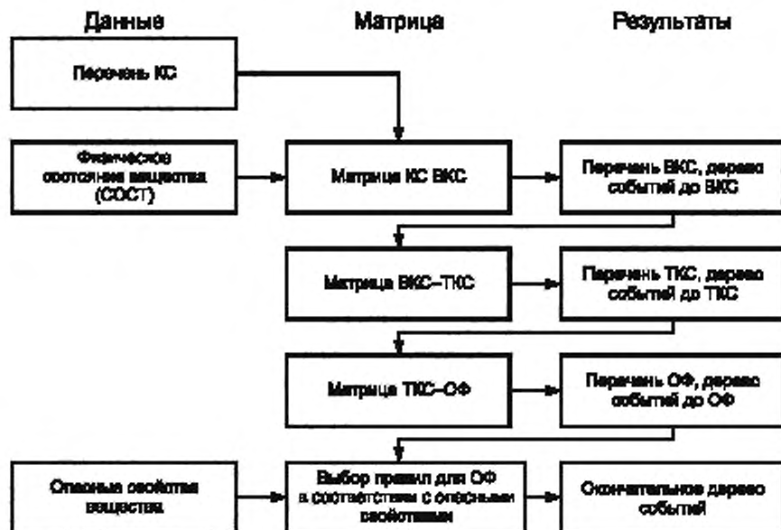
Рисунок 4 — Схема шагов построения дерева событий
