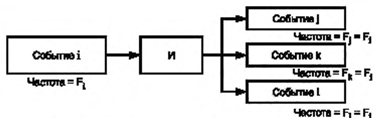
Рисунок 6 — Частота наступления каждого опасного события (ворота «И»)
