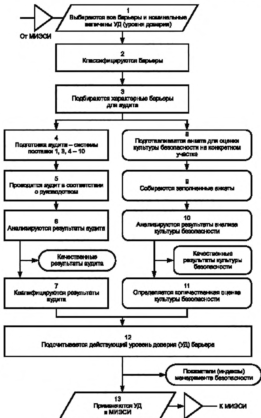
Рисунок 13 — Блок-схема оценки менеджмента безопасности
