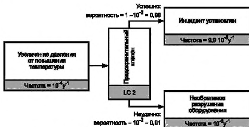
Рисунок 4 — Вероятность наступления событий в развернутом виде
