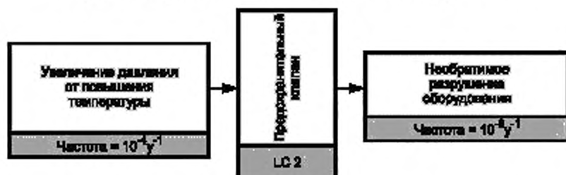
Рисунок 5 — Вероятность наступления событий в упрощенном виде
