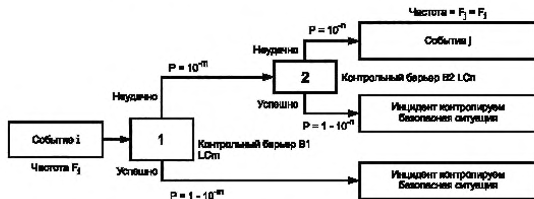
Рисунок 8 — Вероятность перехода событий с использованием барьера «Контроль»
