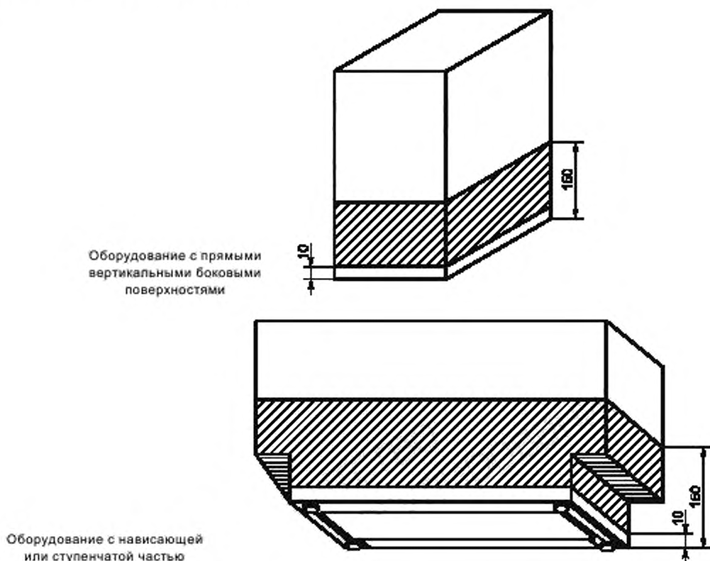
Рисунок 1 — Примеры областей, доступных для пламени свечи
