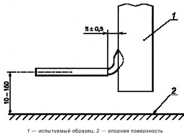
Рисунок 2 — Положение горелки с игольчатым пламенем
