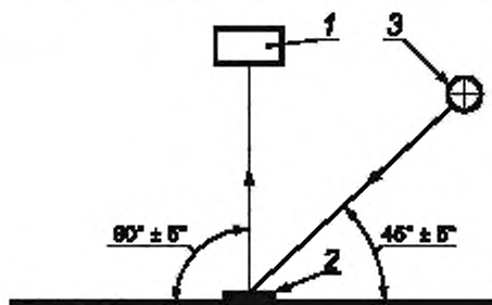
Рисунок 4 — Условия измерения координат цветности и коэффициента яркости
