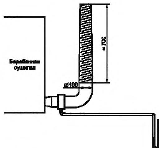
Рисунок А.2 — Стандартное выпускное имитирующее устройство
