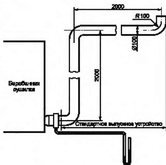
Рисунок А.1 — Стандартное выпускное устройство
