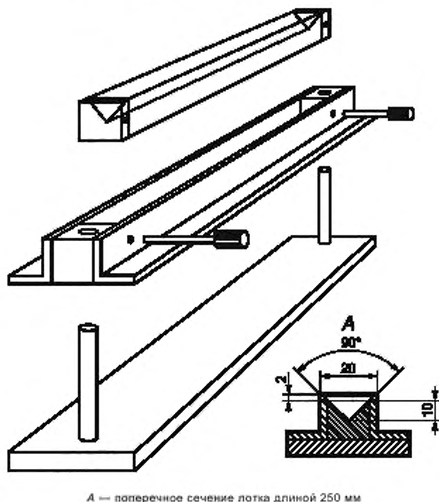
Рисунок 2 — Лоток и приспособления для подготовки образца к проведению испытания воспламеняющейся твердой химической продукции на скорость горения
