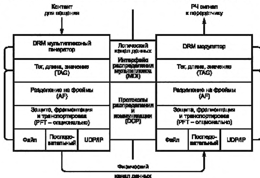
Рисунок 1 — MDI и стек протокола DCP
