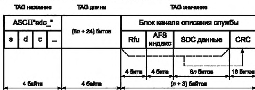
Рисунок 6 — Канал описания служб
