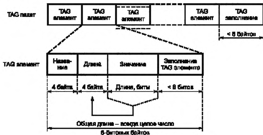
Рисунок 2 — Структура TAG пакета и TAG элемента
