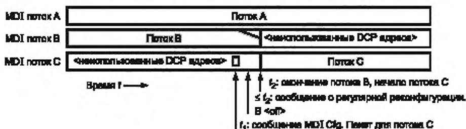
Рисунок Г.2 — Передача двух параллельных MDI потоков
