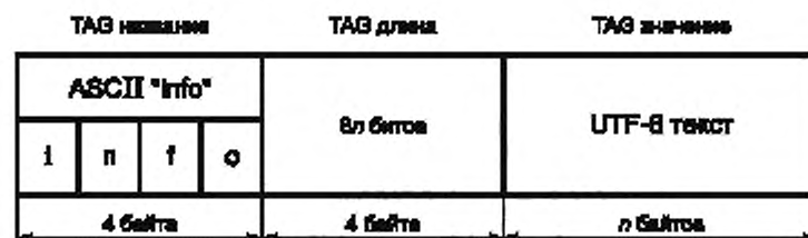
Рисунок 10 — TAG элемент – информация
