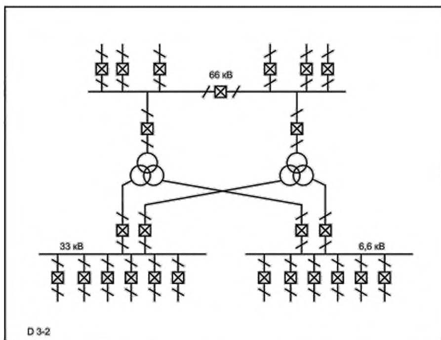
Рисунок А.3 — Примеры типовой однолинейной схемы подстанции типа Д 3
