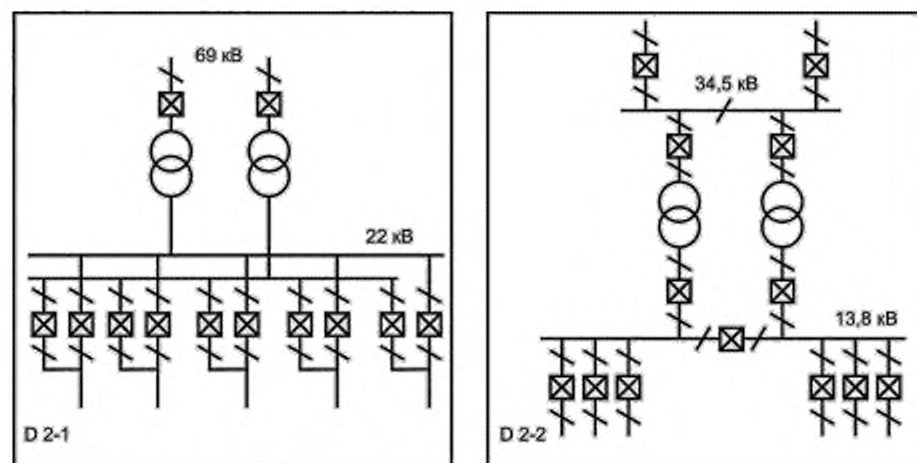
Рисунок А.2 — Примеры типовых однолинейных схем подстанций типа D 2
