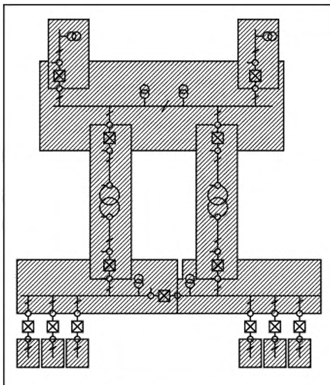
Рисунок А.8 — Типовые зоны защиты
