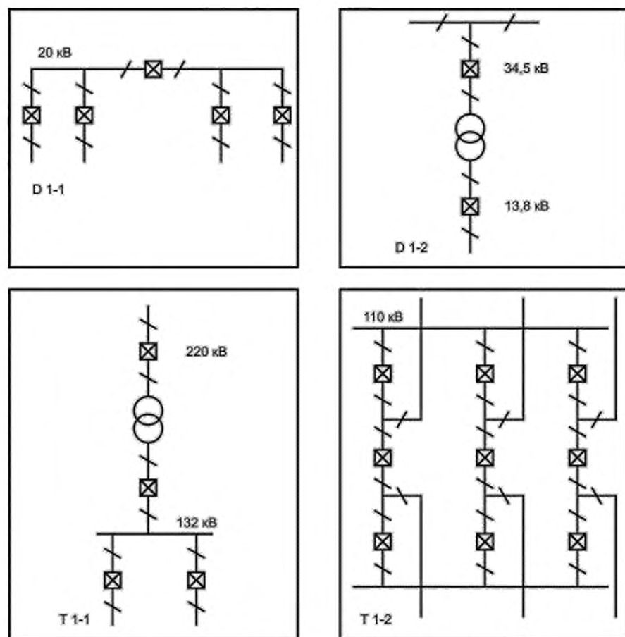
Рисунок 4 — Типы подстанций СН и ВН
