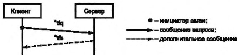
Рисунок E.3 — Транзакция выборки
