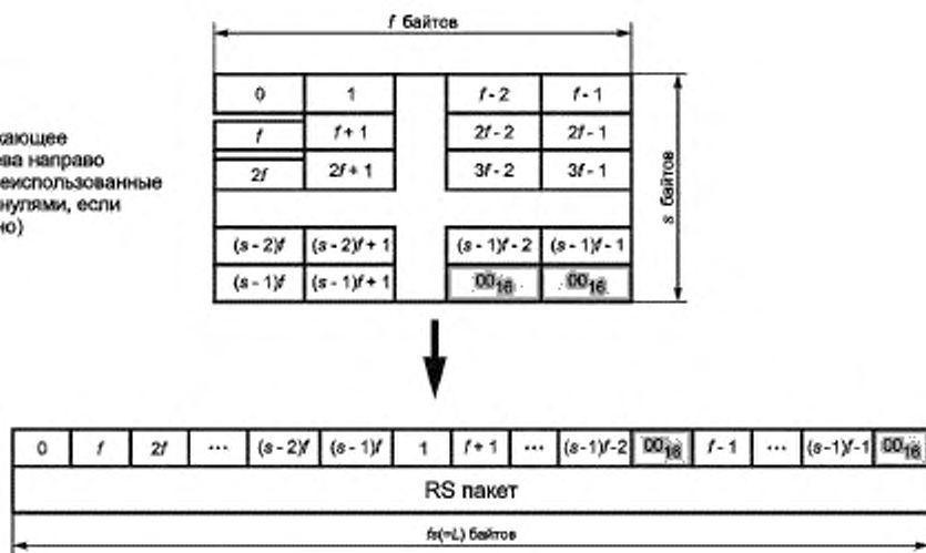
Рисунок 12 — Формирование пакета Рида-Соломона
