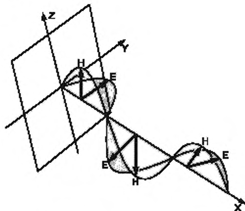
Рисунок 1 — Электромагнитное поле
