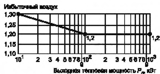
Рисунок 2 — Требования к коэффициенту избытка воздуха
