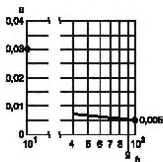
Рисунок 5 — Потери на холостом ходу
