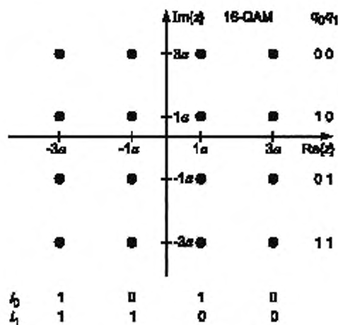
Рисунок 5 — SM 16-QAM отображение с соответствующей битовой комбинацией
