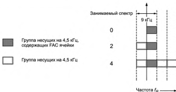
Рисунок 7 — Занимаемый спектр для 9 кГц каналов
