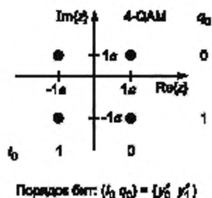
Рисунок 6 — SM 4-QAM отображение с соответствующей битовой комбинацией
