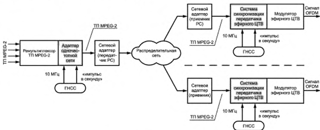
Рисунок 1 — Структурная схема ОЧС
