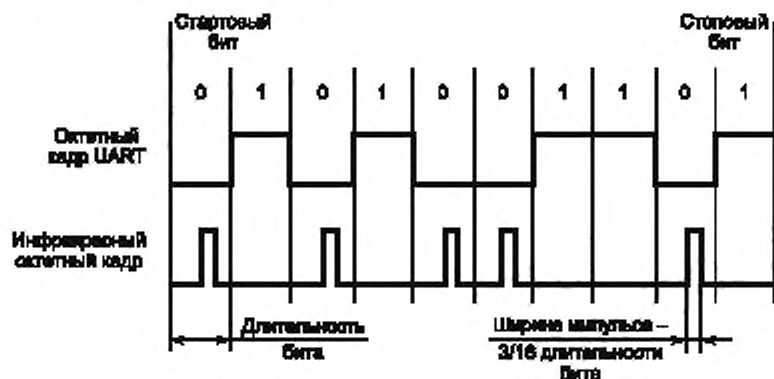
Рисунок А.2 — Кодирование данных 3/16 для IrDA SIR
