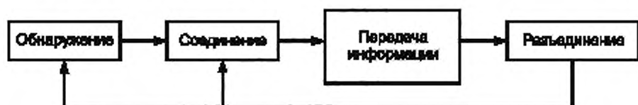
Рисунок 6 — Модуль процедур при обмене данными по IrDA
