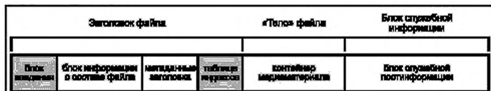
Рисунок П.1 — Основные компоненты простого MXF-файла
