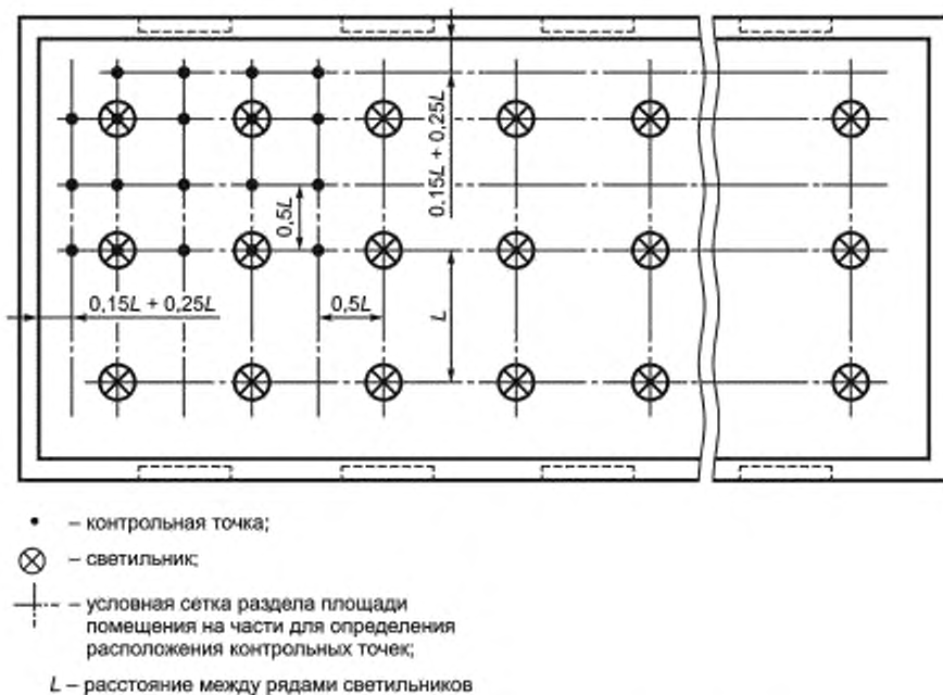
Рисунок А.1 — Расположение контрольных точек при измерении минимальной освещенности помещения от светильников, принимаемых за точечные излучатели
