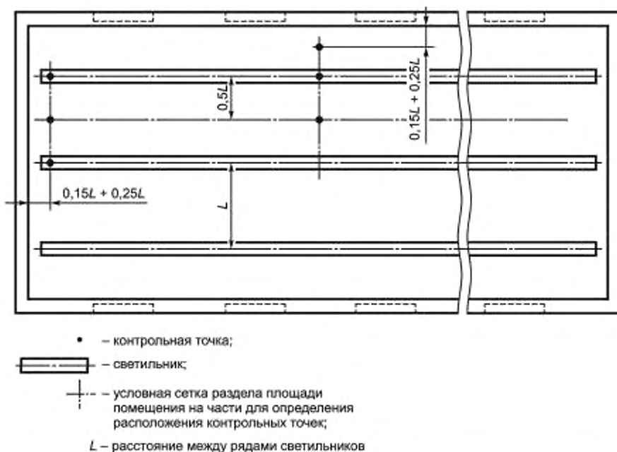
Рисунок А.2 — Расположение контрольных точек при измерении минимальной освещенности помещения от светильников, принимаемых за линейные излучатели
