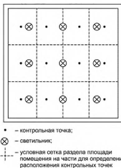
Рисунок А.3 — Расположение контрольных точек при измерении средней освещенности в помещении
