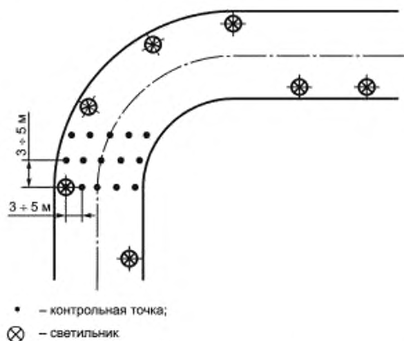
Рисунок А.7 — Расположение контрольных точек при измерении средней освещенности улиц в местах закругления
