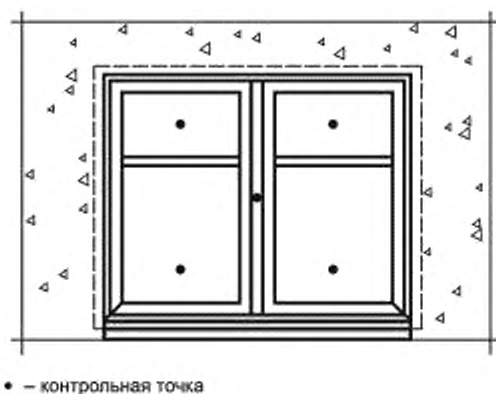
Рисунок А.8 — Расположение контрольных точек на внешней поверхности окна при измерении вертикальной освещенности (уровня засветки окон)
