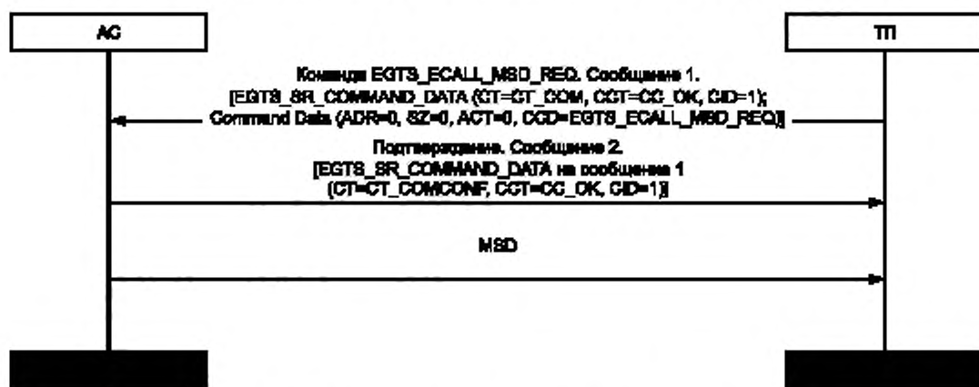
Рисунок 7а — Отправка команды ECTS_ECALL_MSD_REQ по SMS
