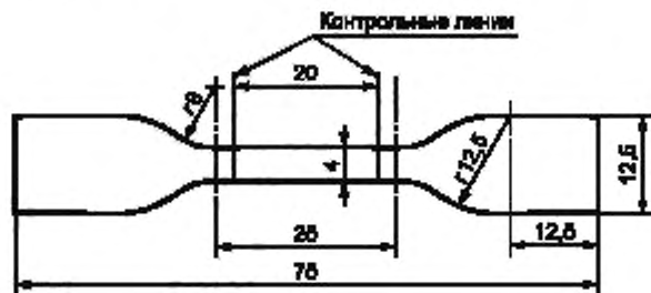
Рисунок 1 — Образец в виде двусторонней лопатки
