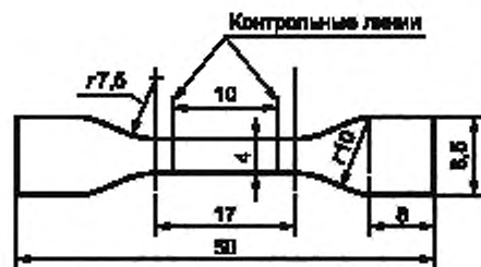
Рисунок 2 — Образец в виде двусторонней лопатки уменьшенного размера
