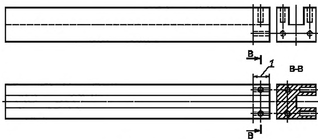
Рисунок 2 — Места отбора проб от подовых блоков, спрессованных с пазом
