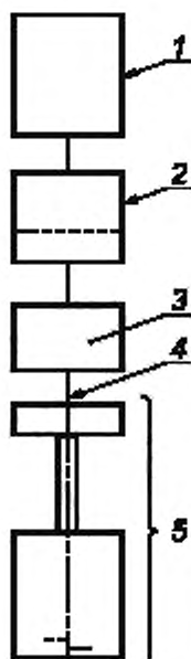
1 — мотор; 2 — муфта сцепления или тормоз; 3 — барабан с делениями или электронный сенсор; 4 — вал; 5 — реторта в сборе
