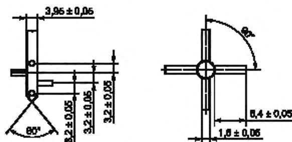
Рисунок 2 — Лопасти металлической мешалки
