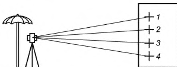
Рисунок 2 — Конфигурация для измерения вертикальных углов
