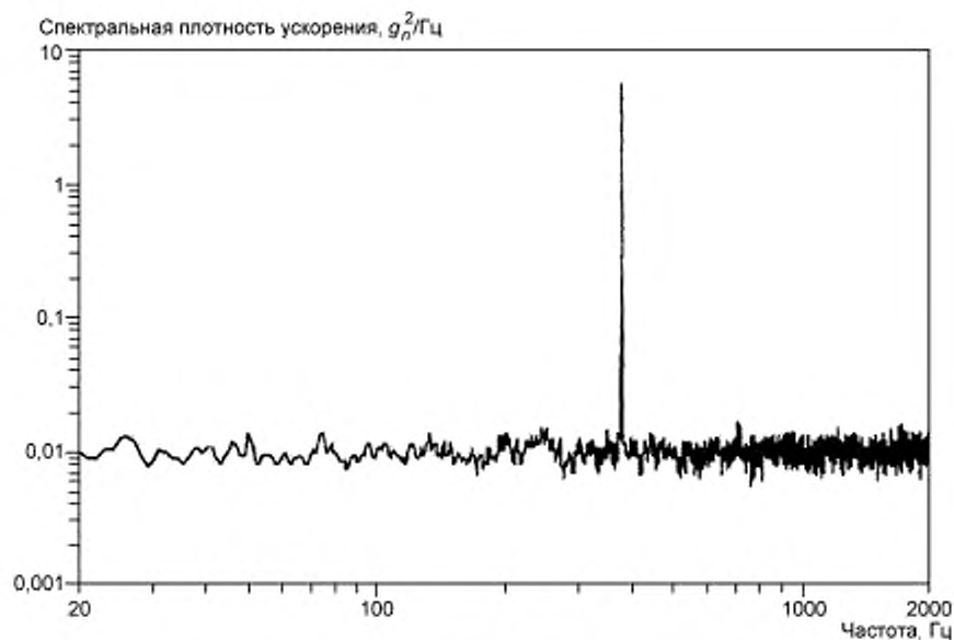
Рисунок А.2 — Гармонический сигнал на частоте 380 Гц
