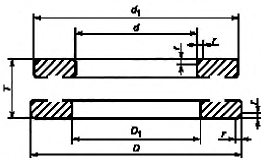
Рисунок 3 — Упорный одинарный и упорно-радиальный подшипник
