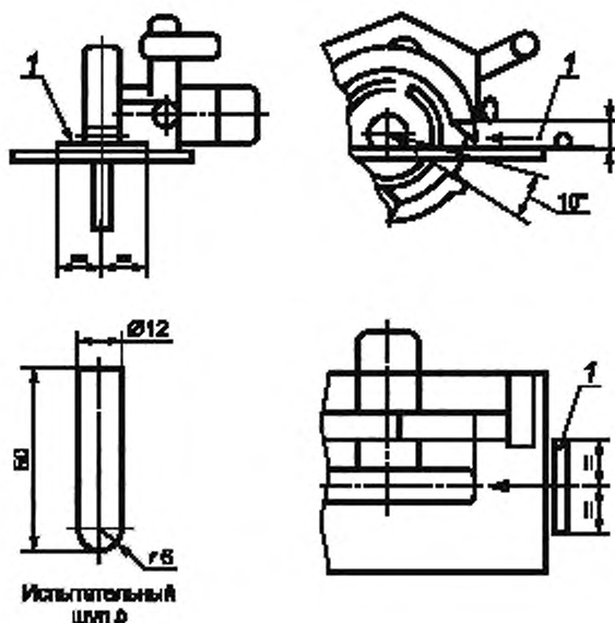
1 — Испытательный щуп «б»
