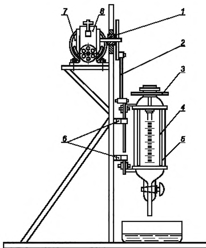
1 — маховик; 2 — шатуны; 3 — зажимное кольцо; 4 — гнездо для делительной воронки; 5 — делительная воронка; 6 — направляющие планки; 7 — электродвигатель; 8 — редуктор
