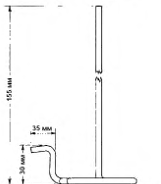
Рисунок 1 – Подающая трубка
