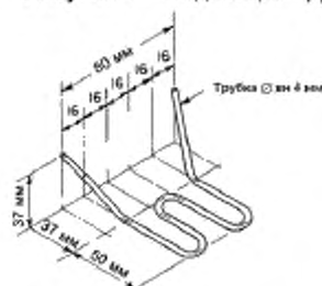
Рисунок 2 – Змеевидная трубка
