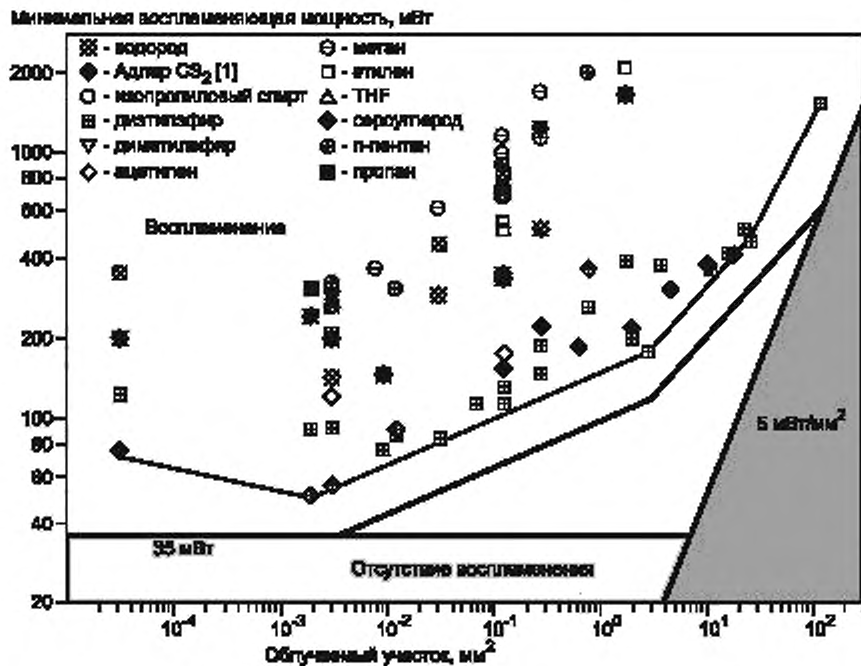
Рисунок 1 — Рисунок В.1 с предельными линиями для промежуточных значений площадей облучаемой поверхности в присутствии негорючих поглотителей (классы температур Т1-Т4, электрооборудование подгрупп IIA, IIB, IIC)
