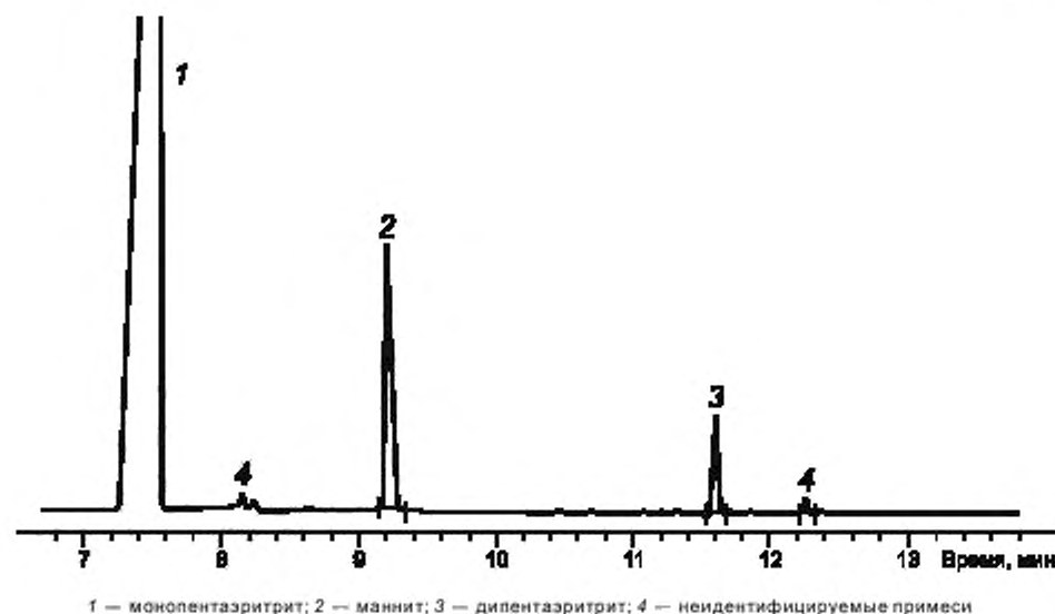
Рисунок 1 — Тиловая хроматограмма технического пентаэритрита
